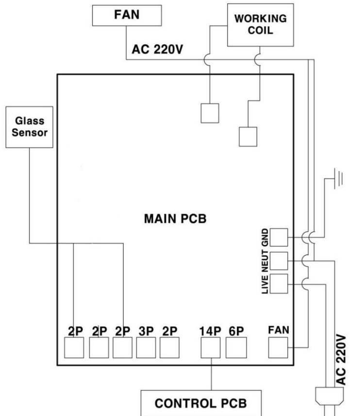
DWU05 Wiring Diagram
